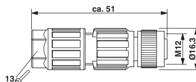
Maßzeichnung
